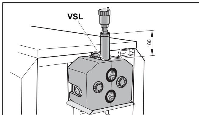
Рис. 54 Установка воздушного клапана на предохранительной подающей линии
