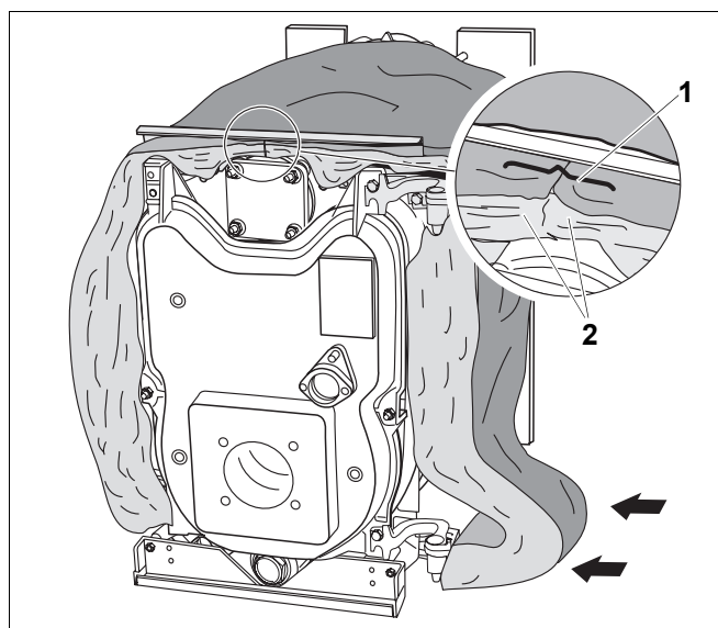
Рис. 39 Монтаж теплоизоляции
