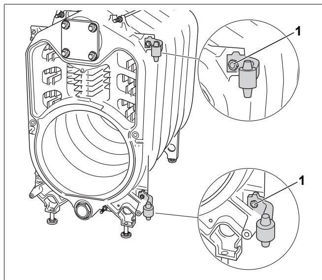
Рис. 33 Монтаж шарнирных крюков (здесь: с правой стороны)
