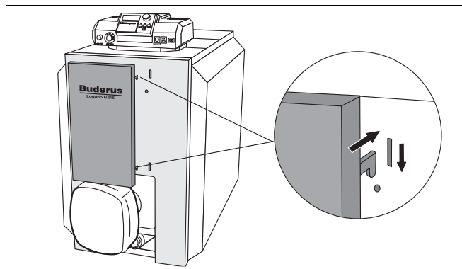
Рис. 70 Монтаж декоративного элемента
