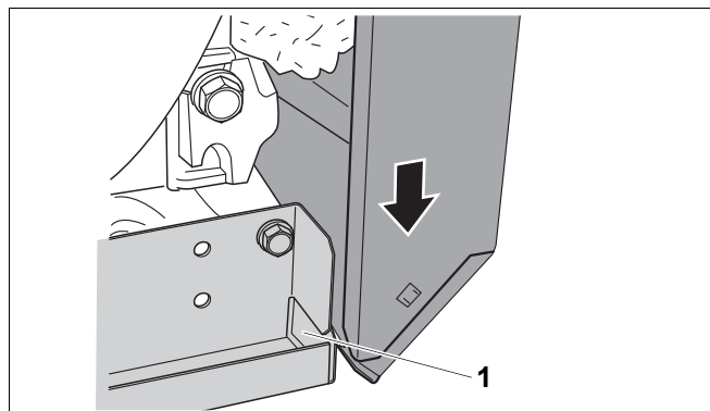
Рис. 42 Установка боковой стенки спереди внизу.
