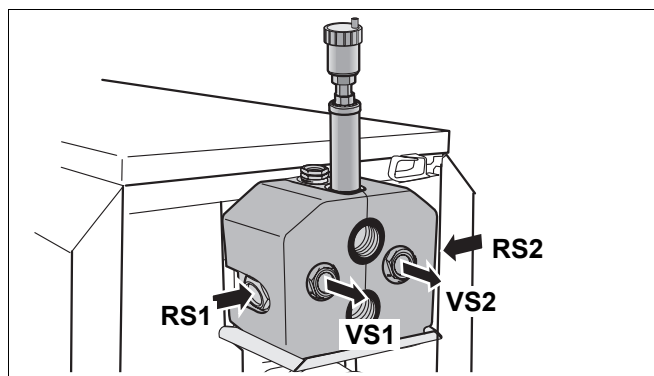
Рис. 55 Подключение бака-водонагревателя
