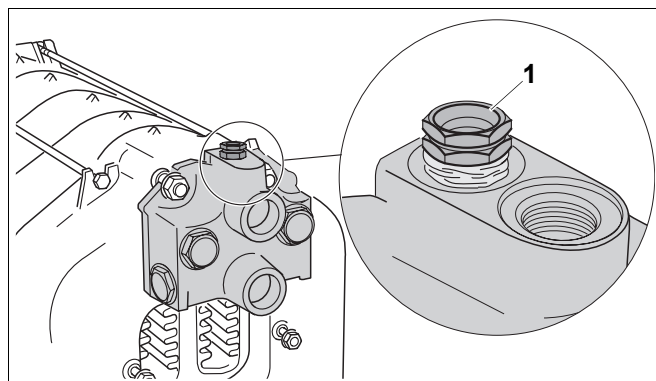
Рис. 29 Установка гильзы для датчиков
